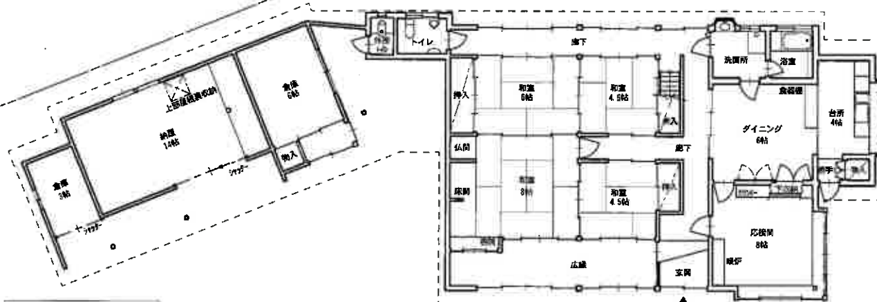
新屋棟 1階平面図 1/200
