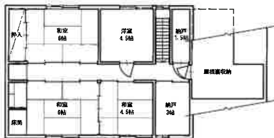
住宅棟 2階平面図 1/200
